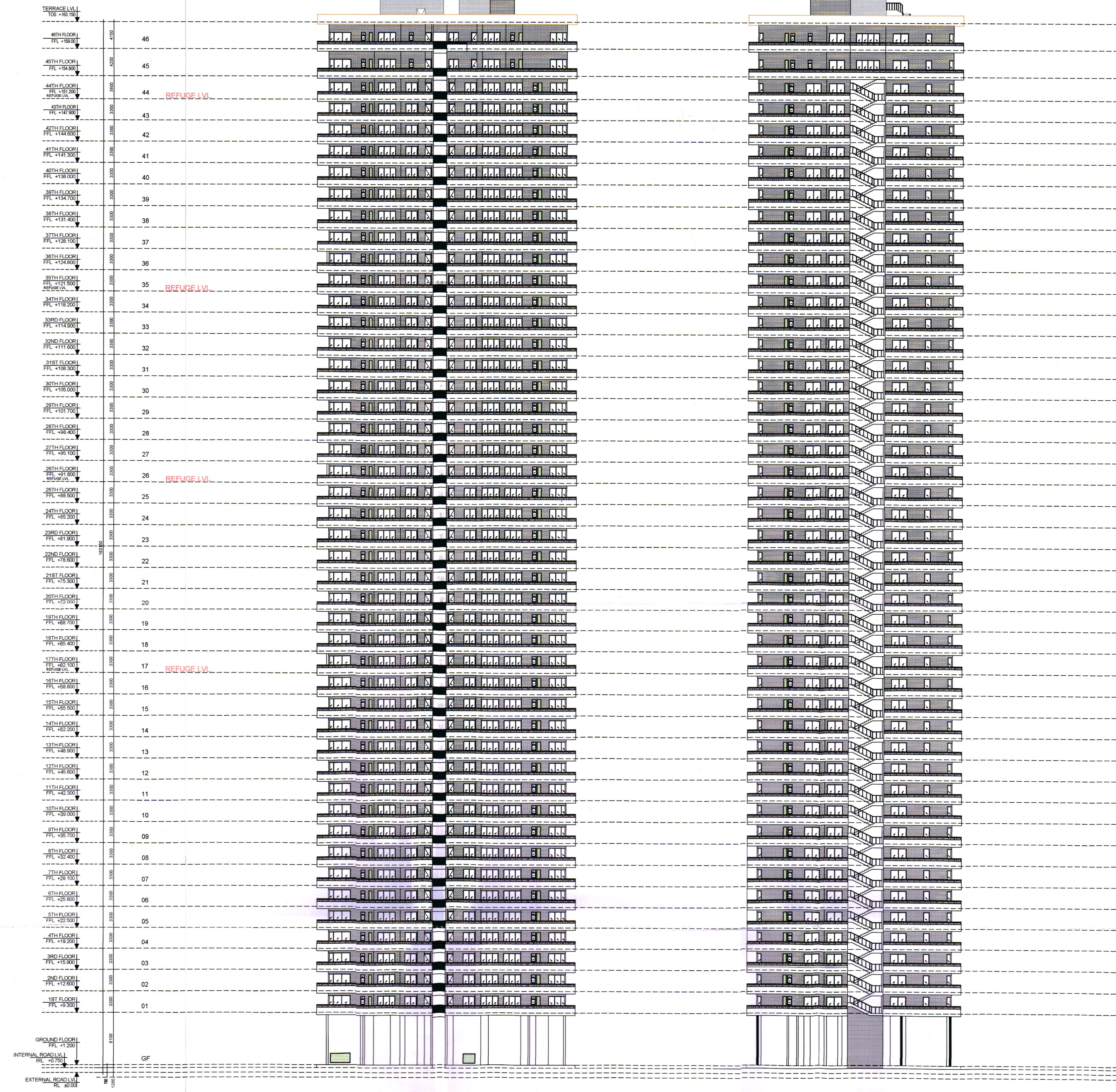
ELEVATION A
