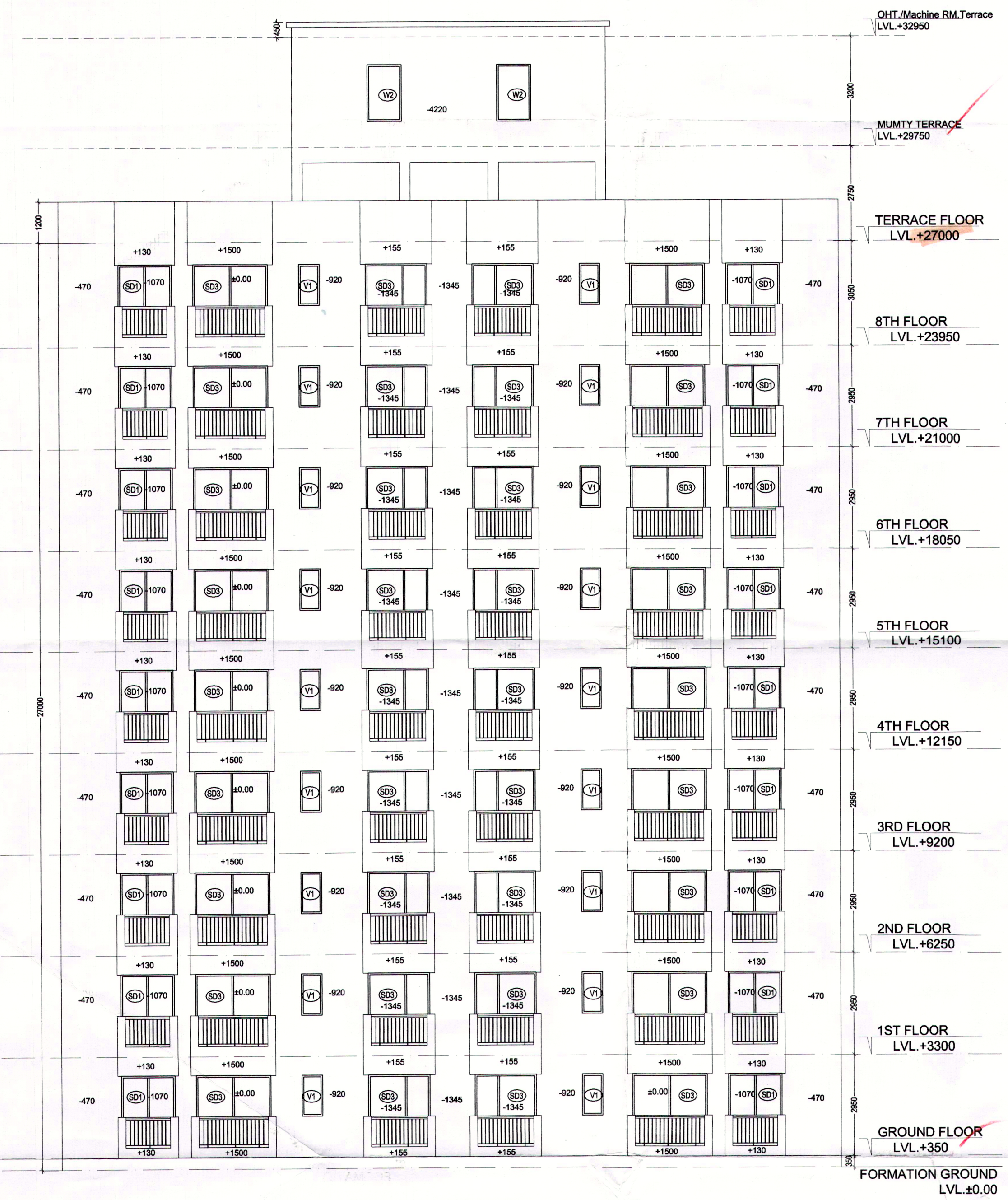
ELEVATION - C
