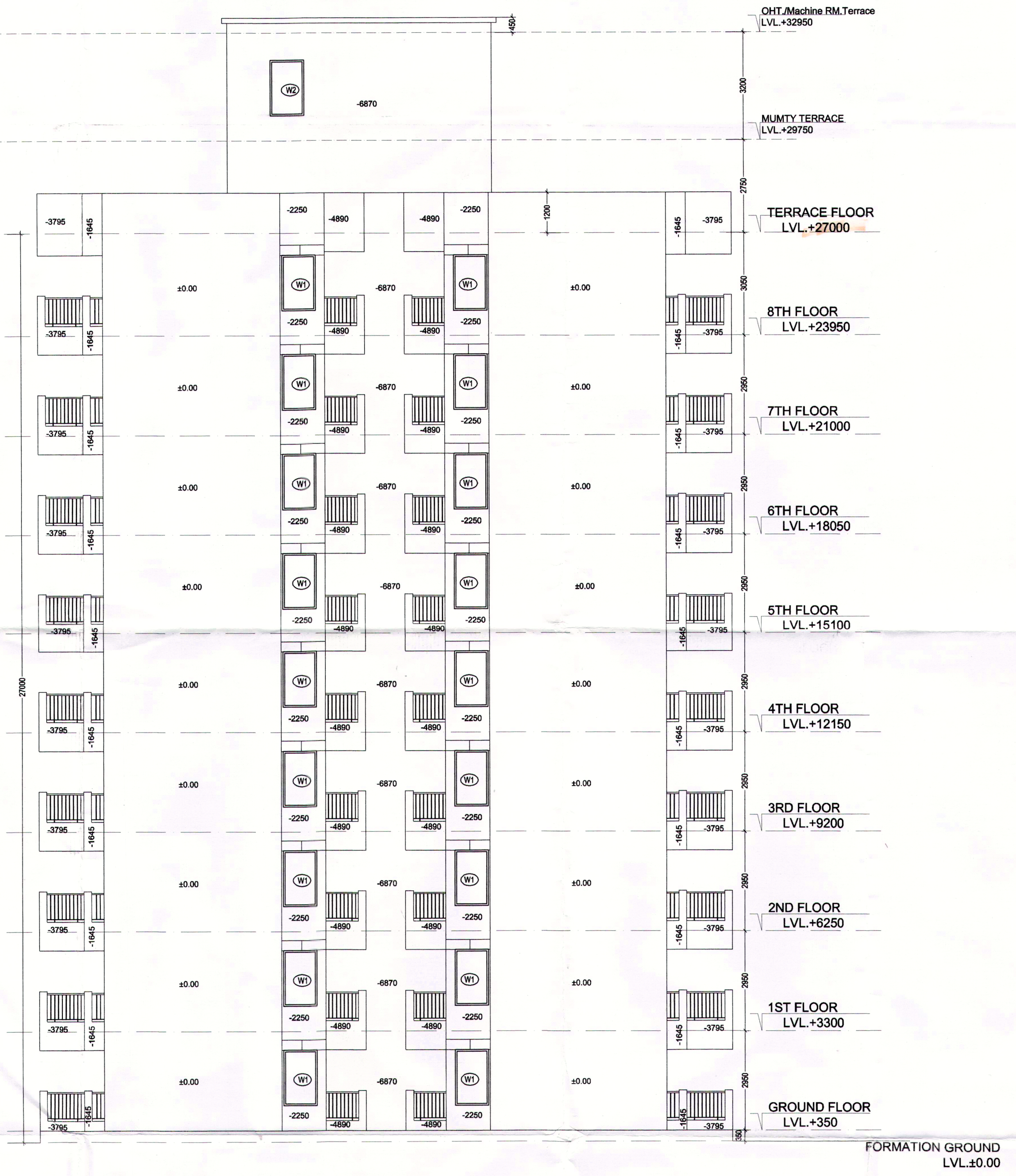
ELEVATION - D
