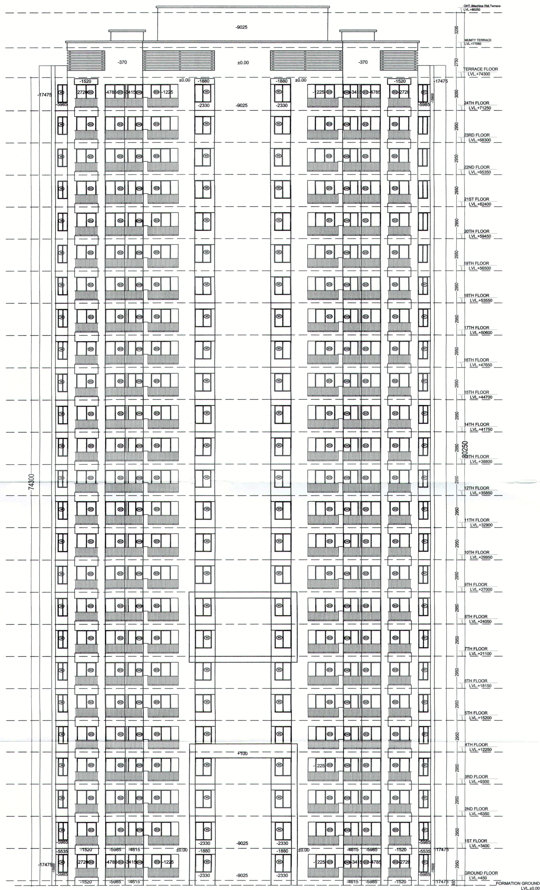
ELEVATION - C
