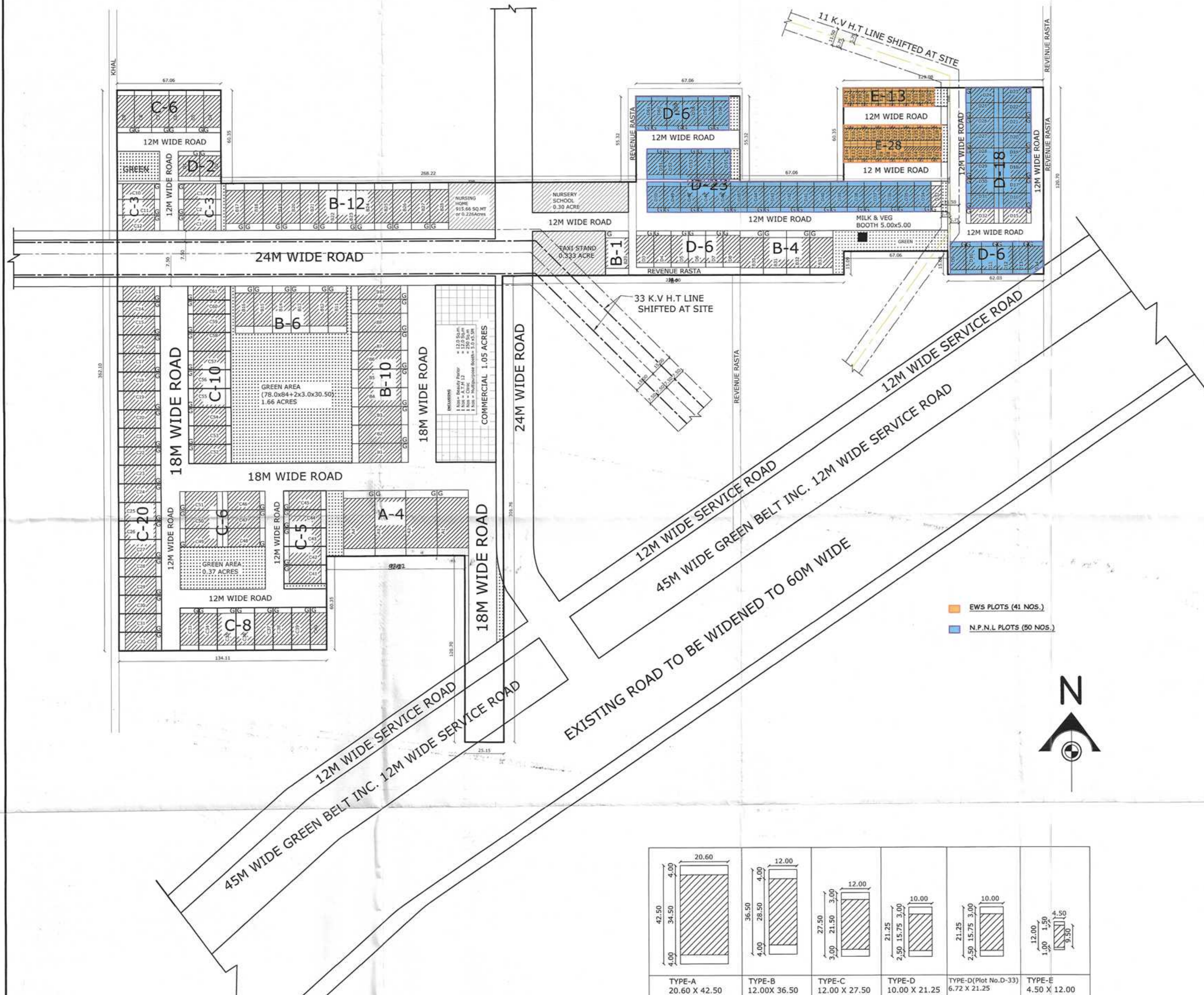
ZONING PLAN SCALE : 1:1000
