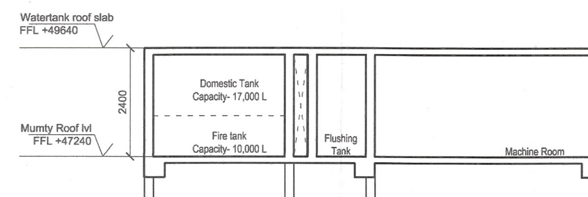
4 OHT Section SCALE - 1:85
