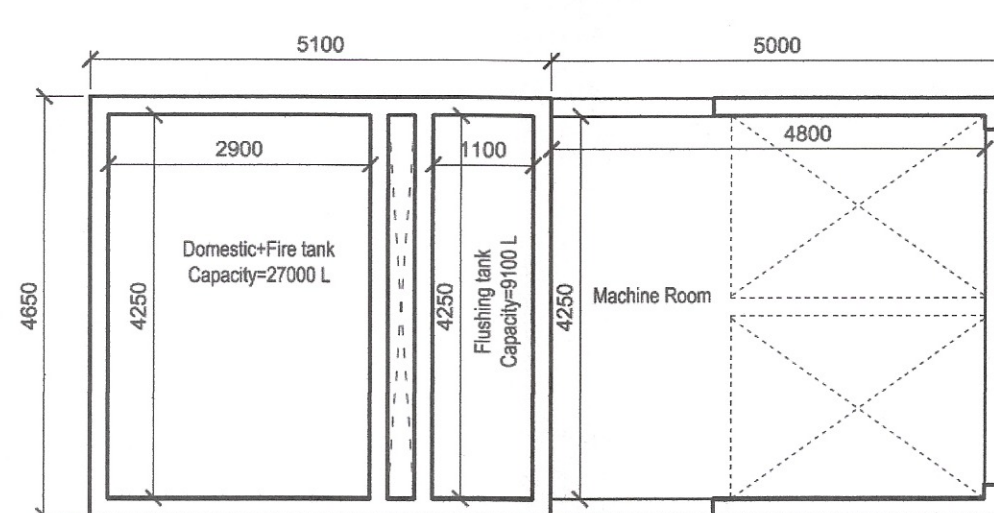
3 OHT Layout (Mumty 02) SCALE - 1:85
