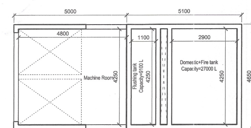
2 OHT Layout (Mumty 01) SCALE - 1:85
