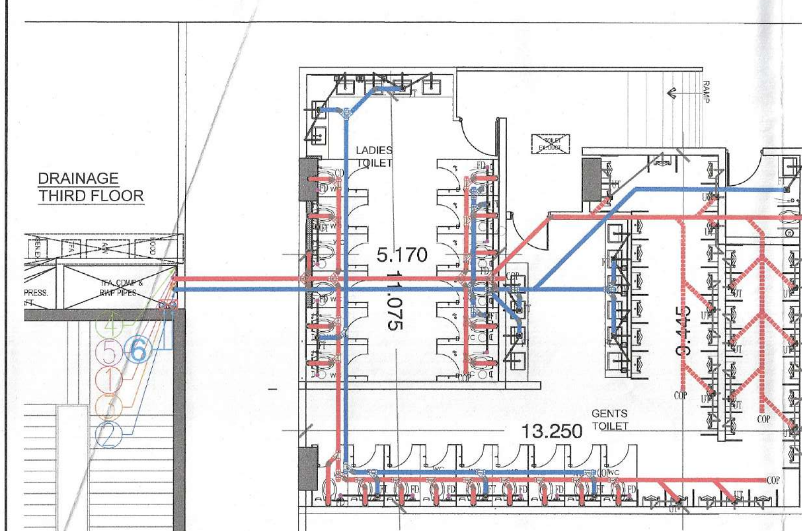
TOILET-3 SCALE - 1:100
