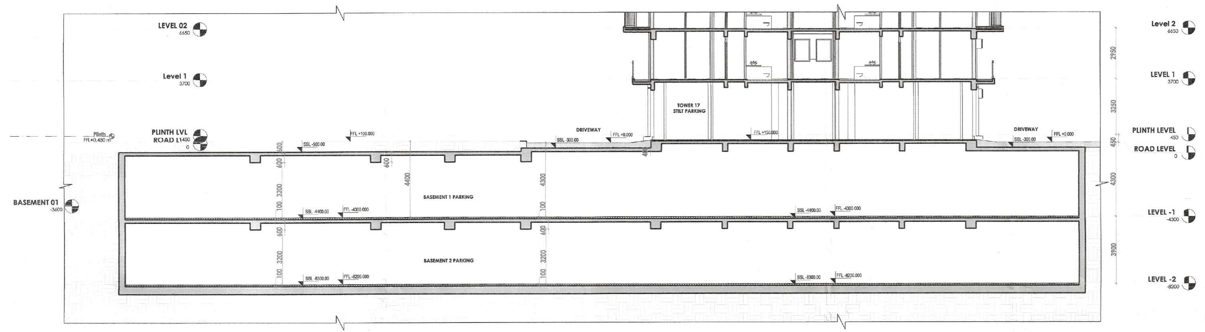
1 Section 35 1:100
