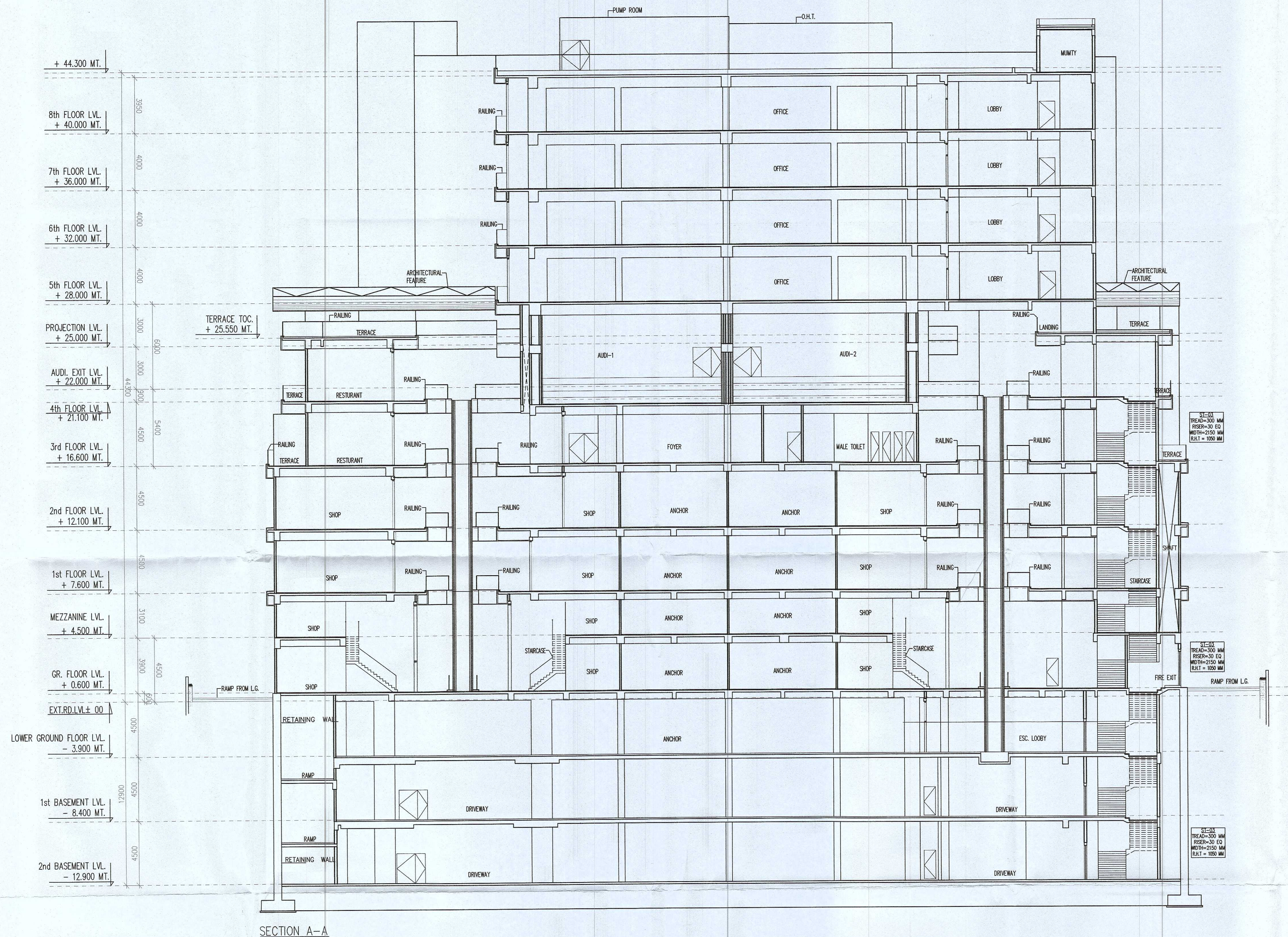
SECTION A-A
