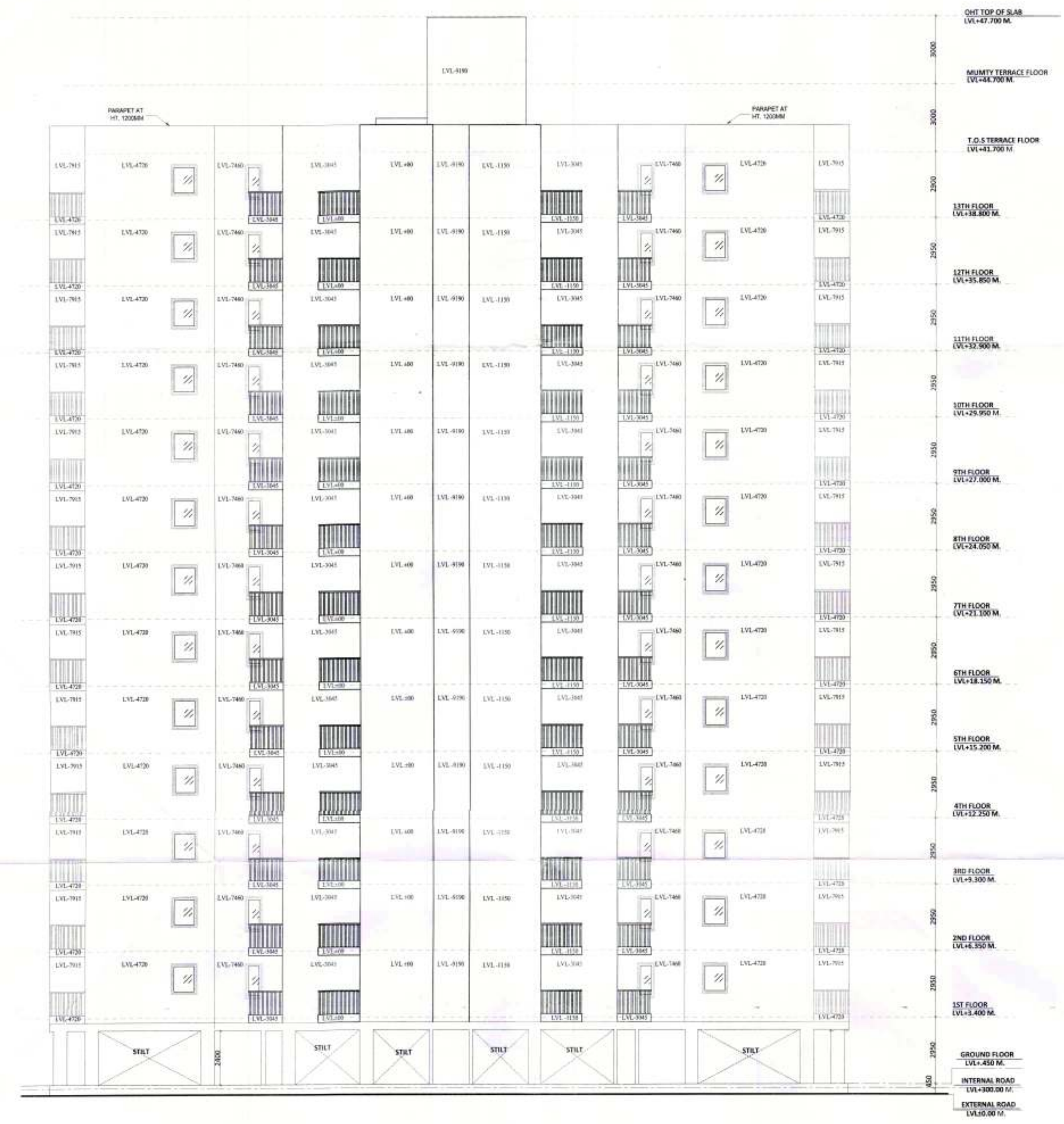
1 ELEVATION E1 Scale: 1:150
