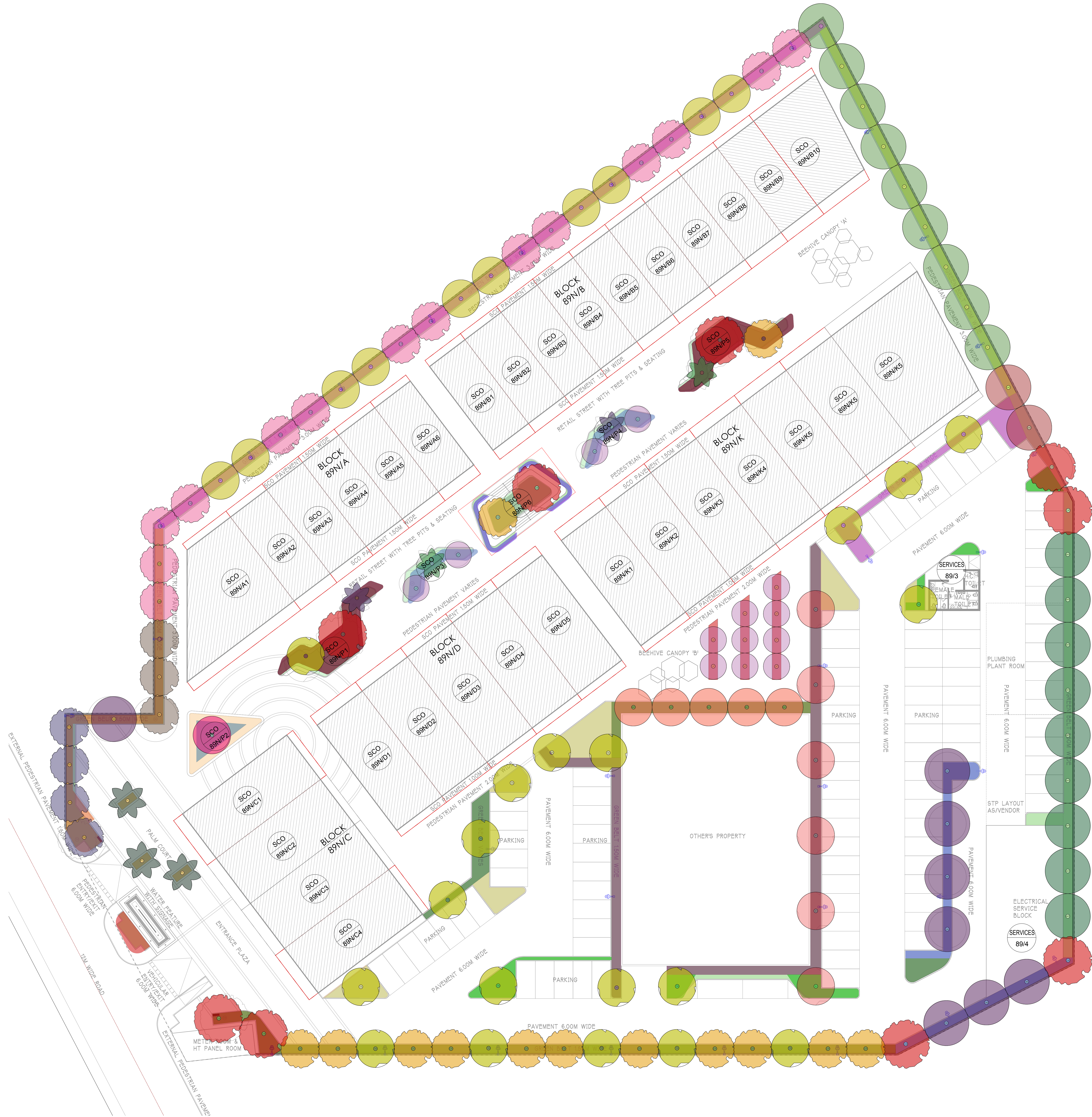
1 PLANTING PLAN PART -02 SCALE: 1:200
