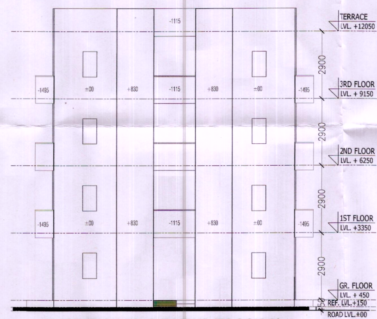
ELEVATION E2 & E4 EWS (BLOCK-A)
