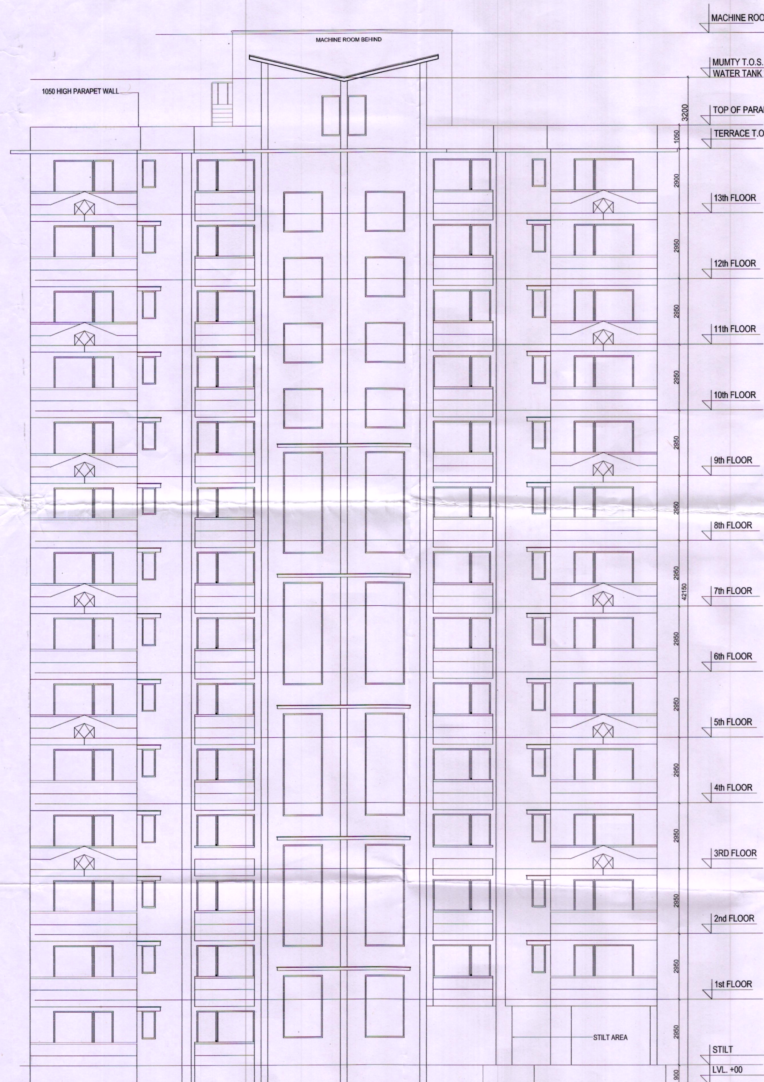
ELEVATION A
