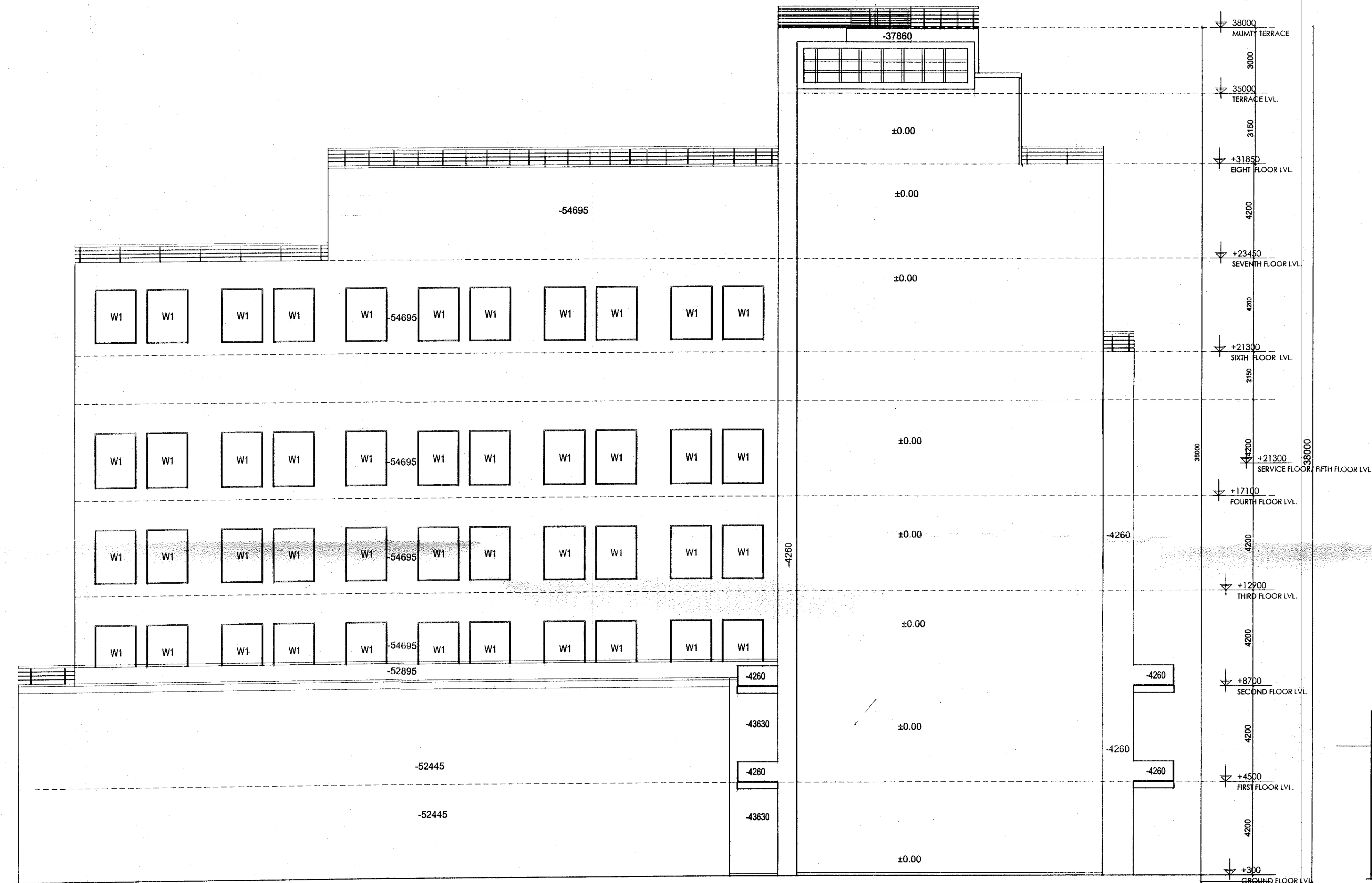
ELEVATION - 'C'
