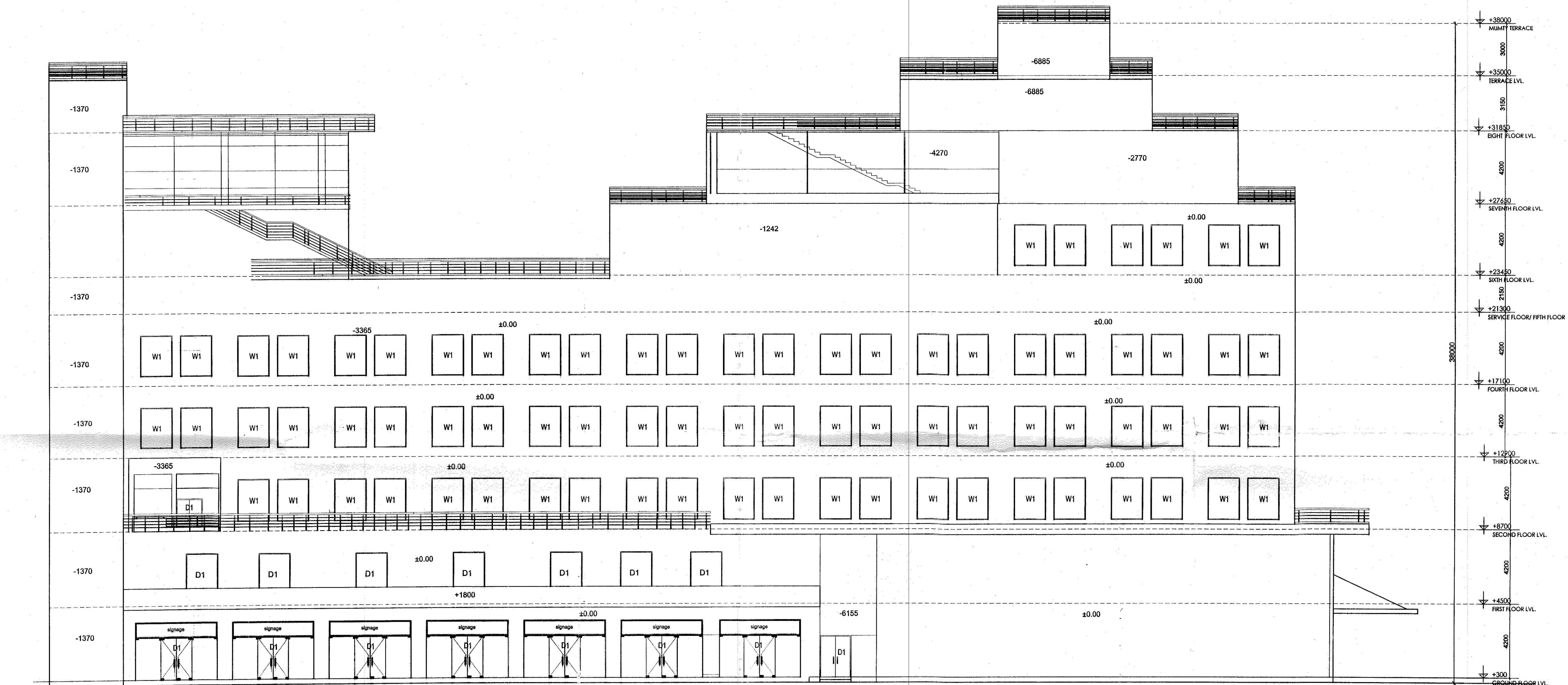
ELEVATION - 'B'
