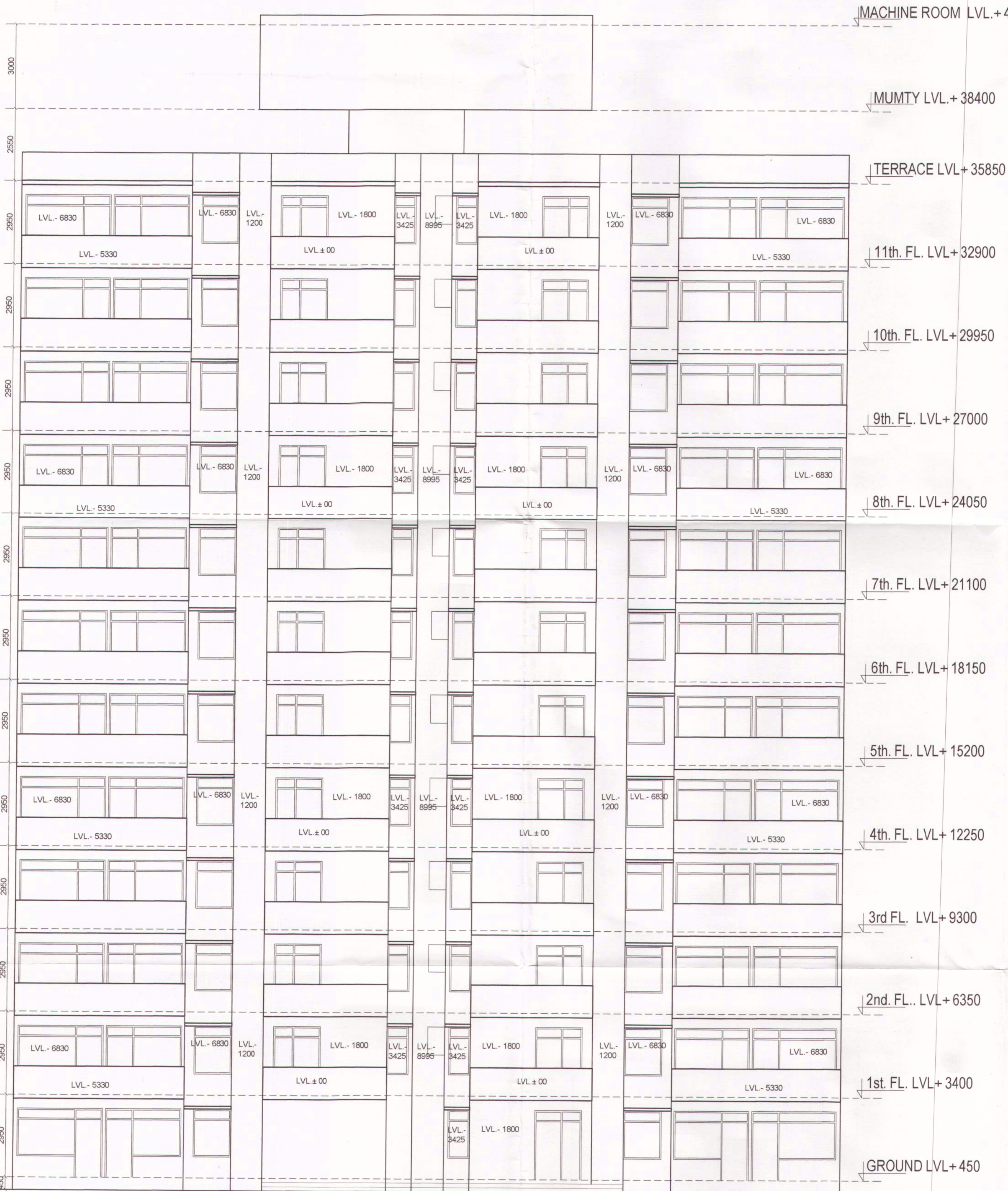
ELEVATION - 1
