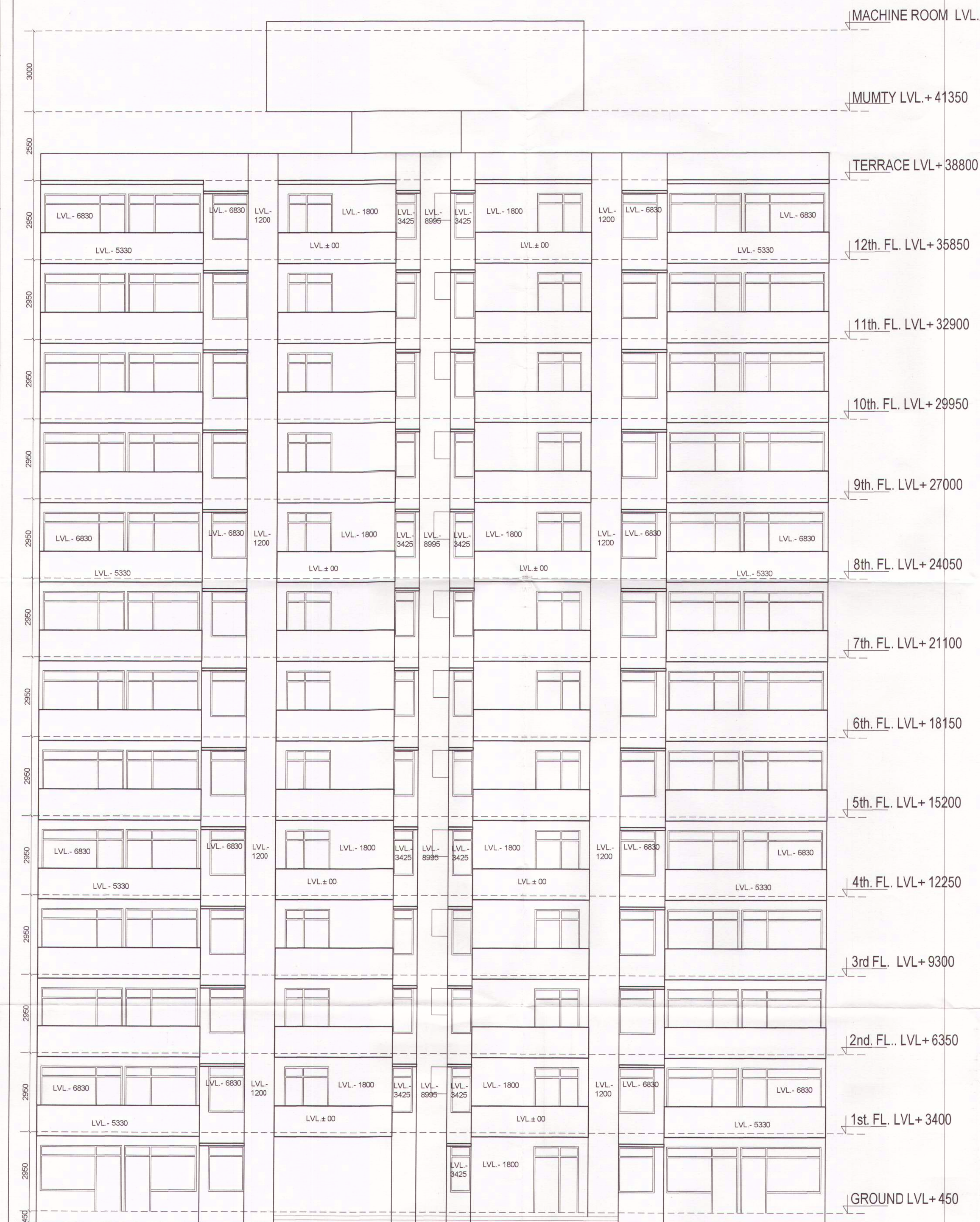
ELEVATION - 1
