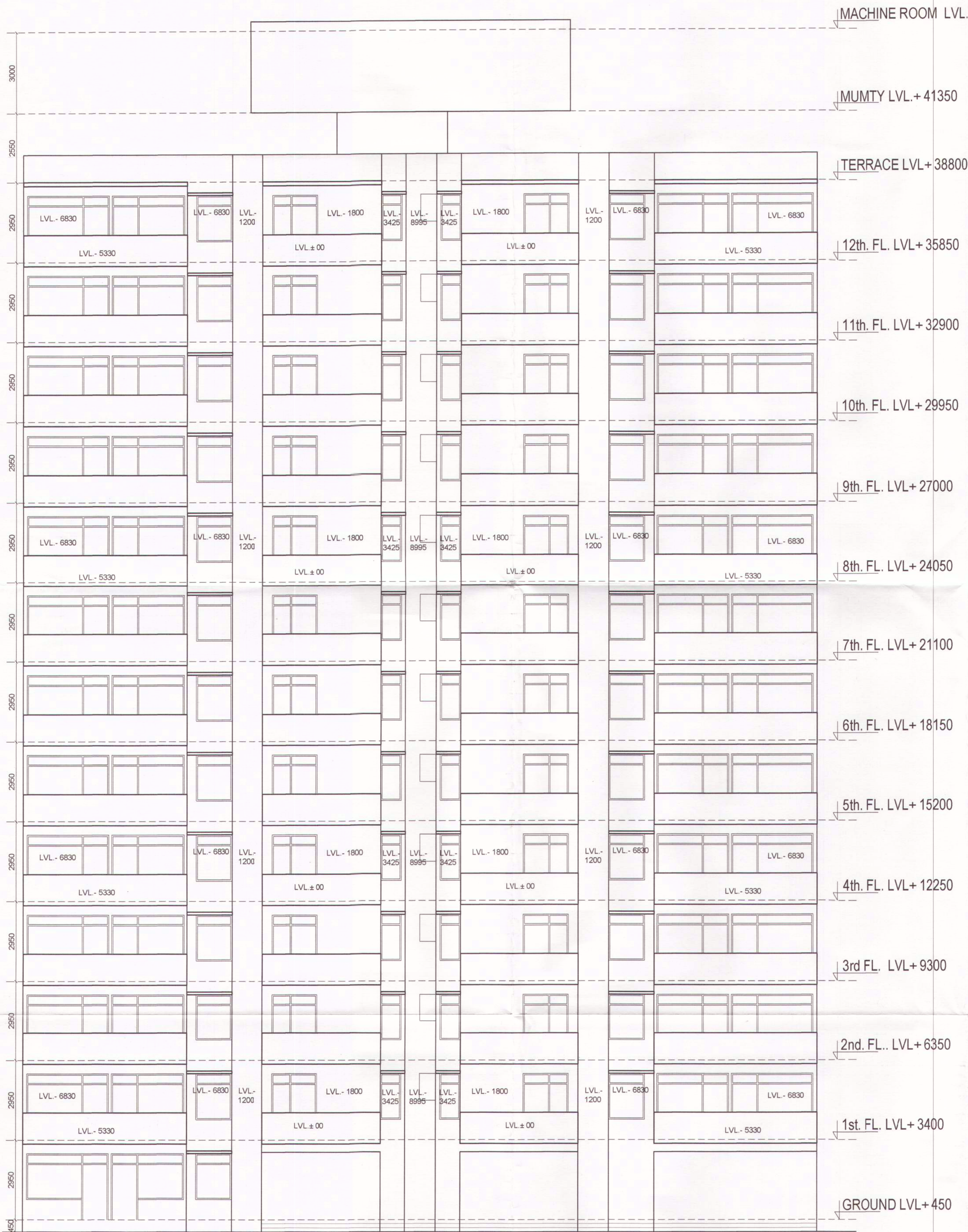
ELEVATION - 1
