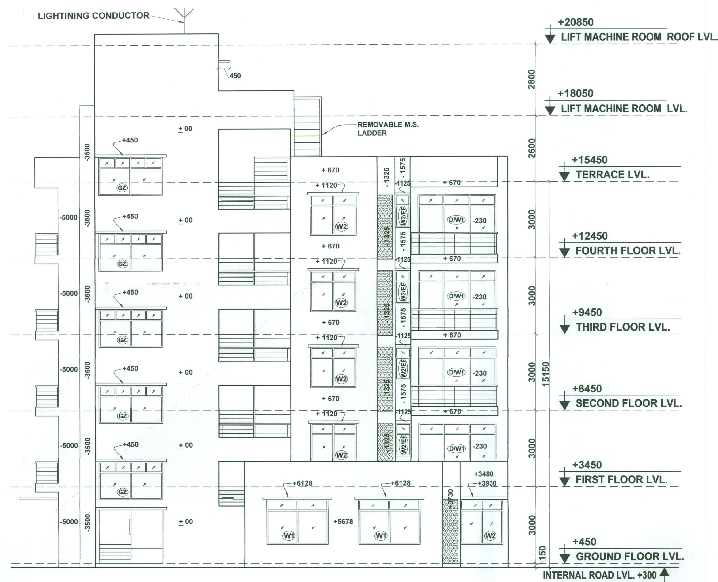
ELEVATION - A
