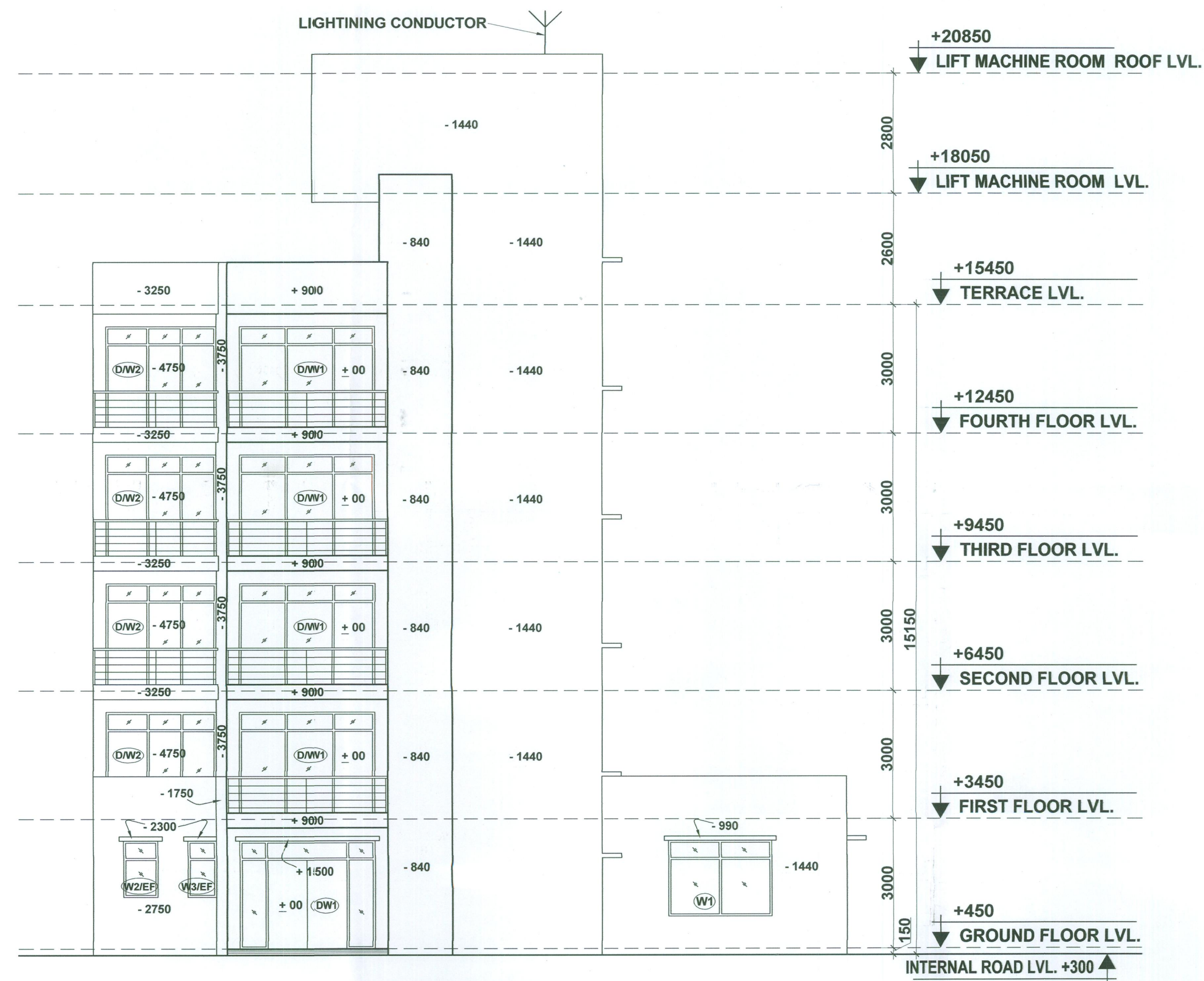
ELEVATION - B
