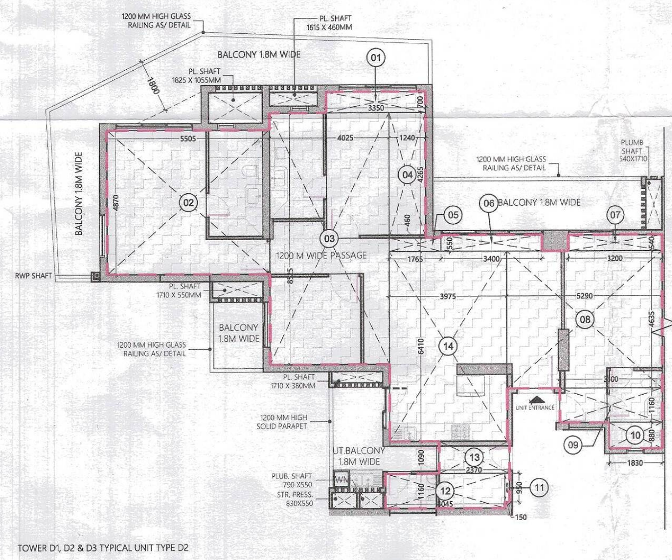
04B TOWER D1, D2 & D3 - TYPICAL UNIT (TYPE D2) REF: SCALE: 1:100
